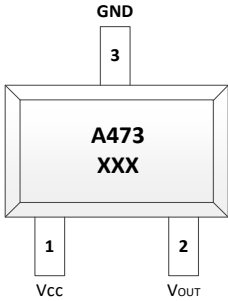
SOT23-3L
